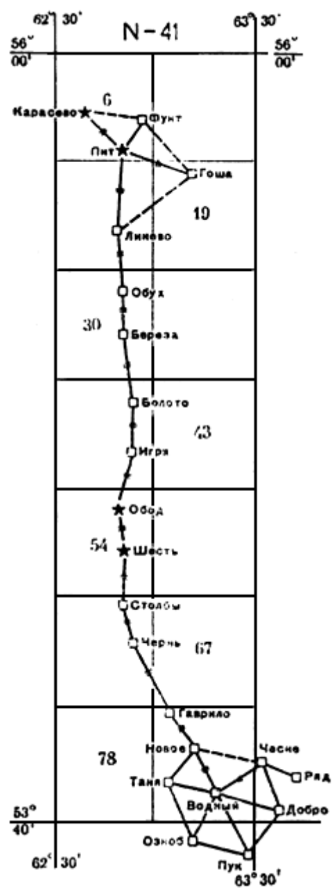
Схема звена полигонометрии 1 класса Карасево-водный
