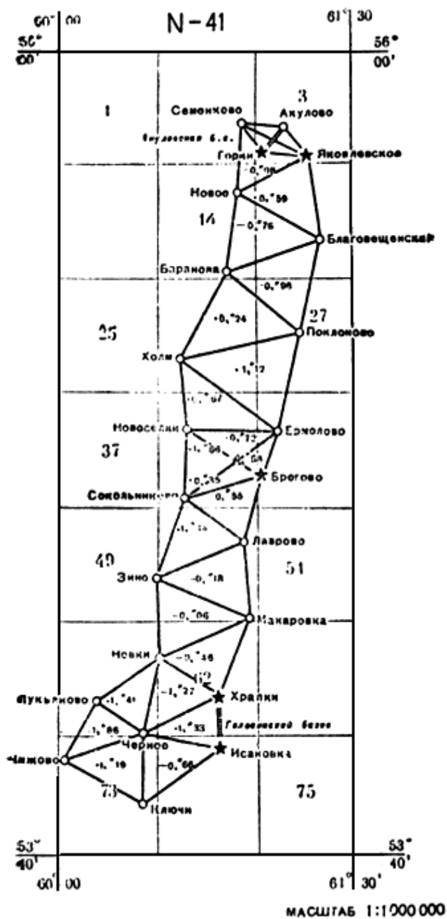
Схема звена триангуляции 1 класса Акулово-Головино
