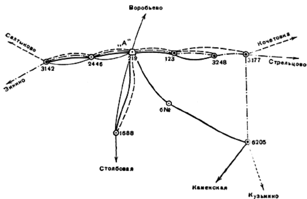
Схема узла связи "А" (фунд. реп. 219)
