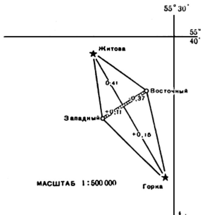
Схема Сергеевской базисной сети
