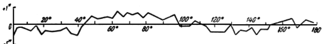
График ошибок диаметров круга триангуляционного теодолита ТТ2"/6" N 8542
